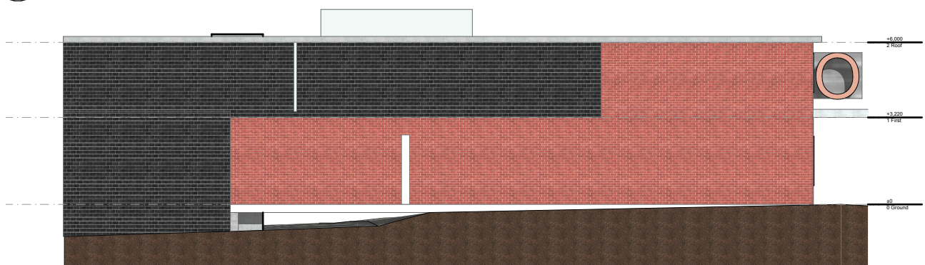
Elevation B-B 1:200
